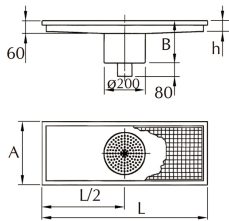
Canales recogeaguas con rejilla serie ECO
