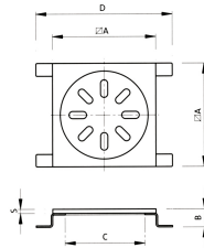
Tapas de registro en acero inoxidable (ligeras)
